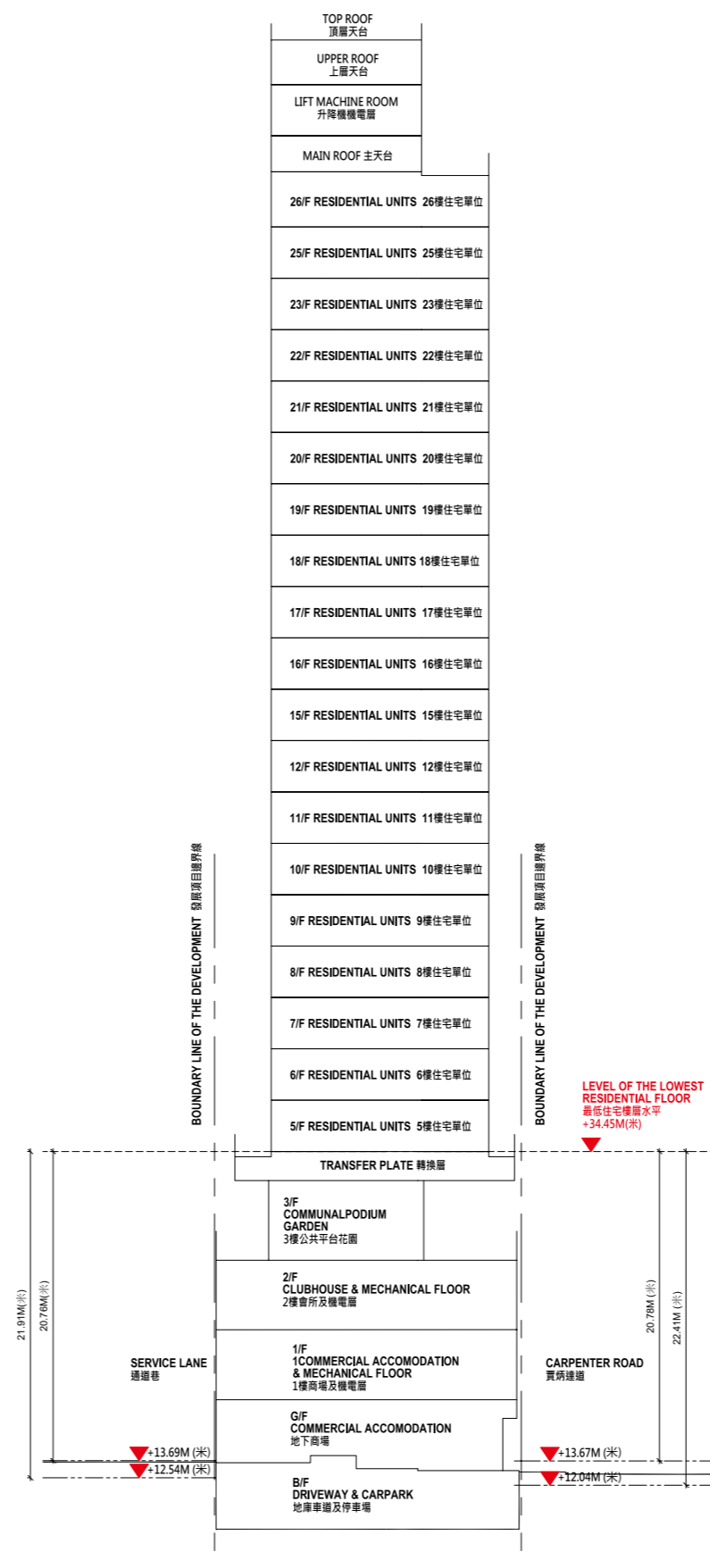
CROSS-SECTION PLAN B-B 橫截面圖 B-B
